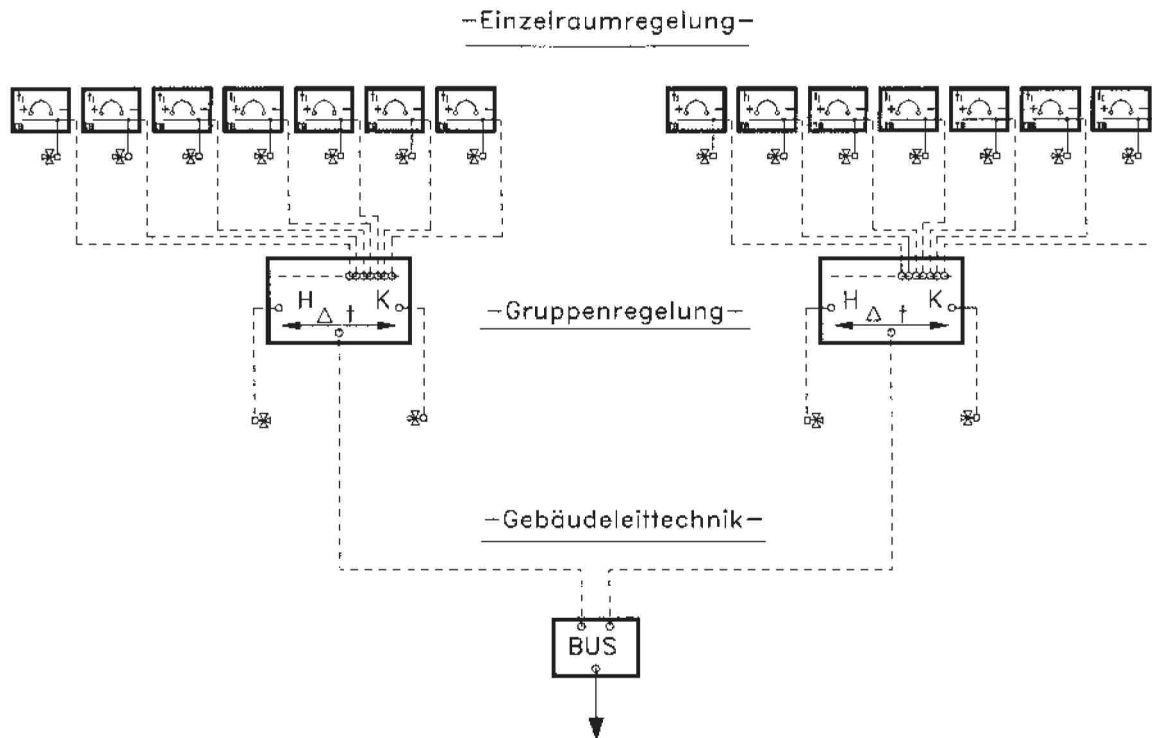
Konzept Regelung
